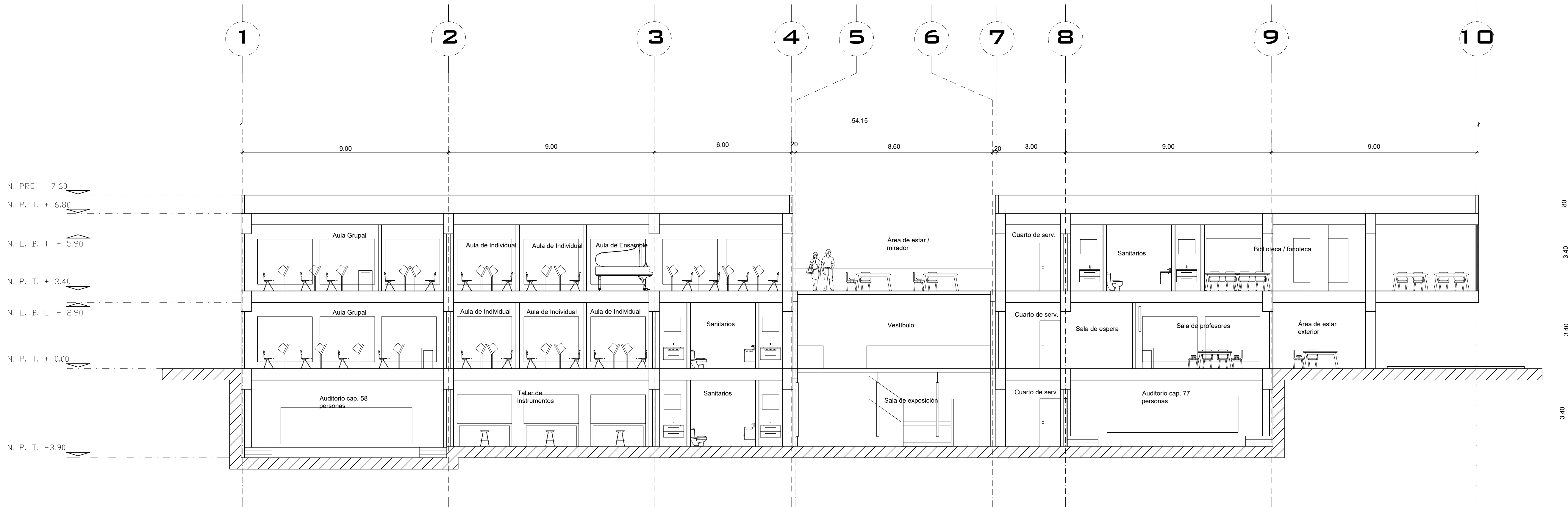
CORTE CC - CC'
