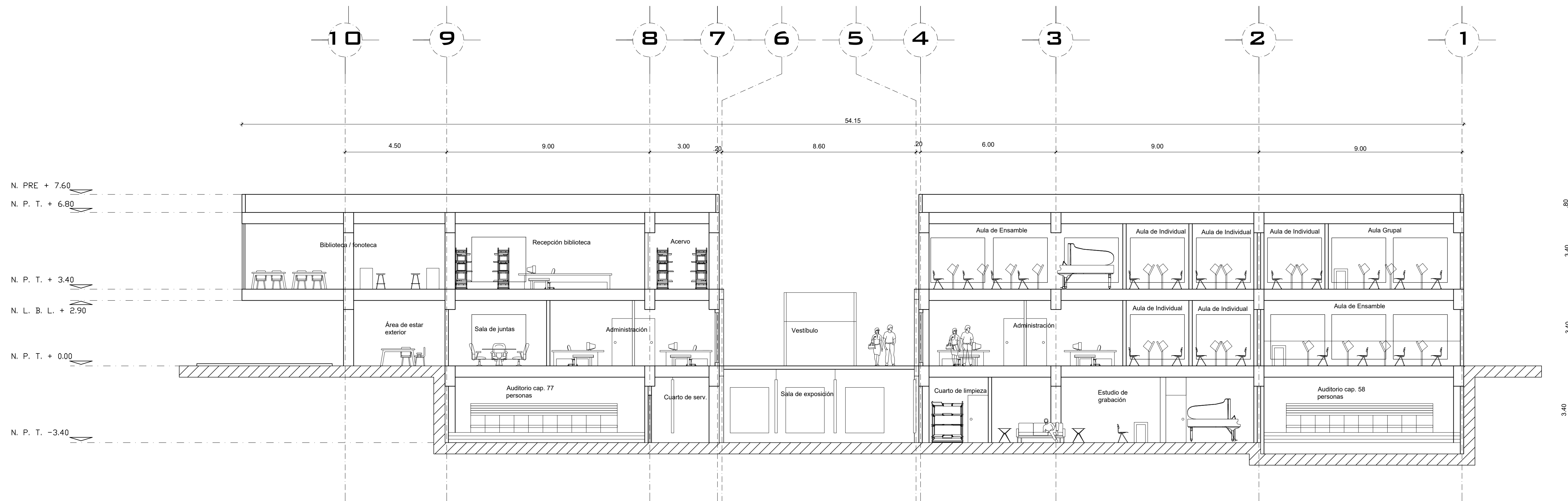
CORTE CD' -CD
