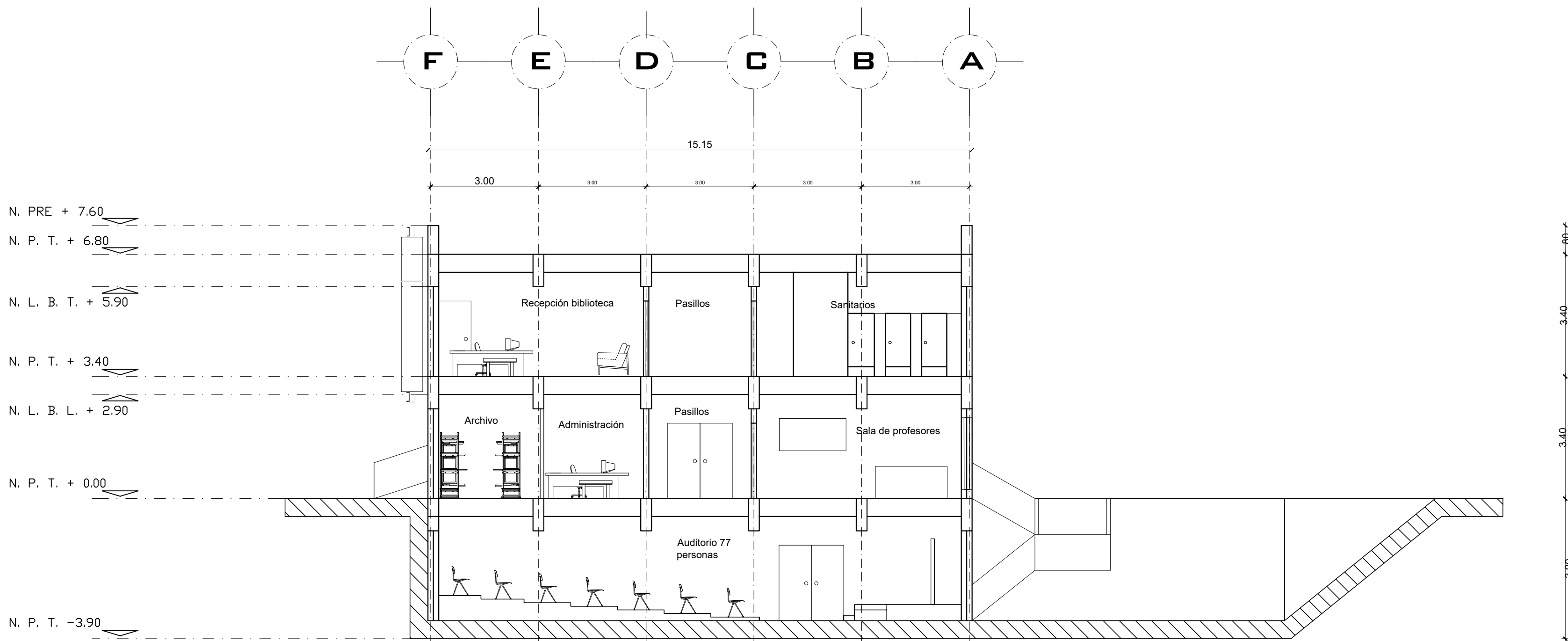
CORTE CB' - CB
